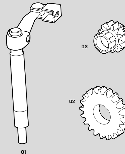
OVLÁDACÍ HŘÍDELKA SPOJKY PUSH ROD
