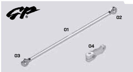
KOMPLETNÍ TÁHLO ŘAZENÍ COMPLETE SHIFT LINKAGE
